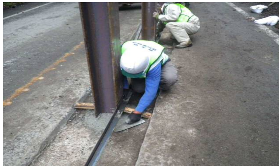
▲ 根固めコンクリート打設状況②
